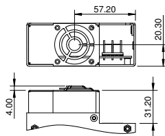
FAN OPTION
